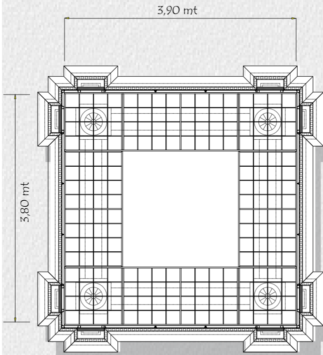
PIANTA
