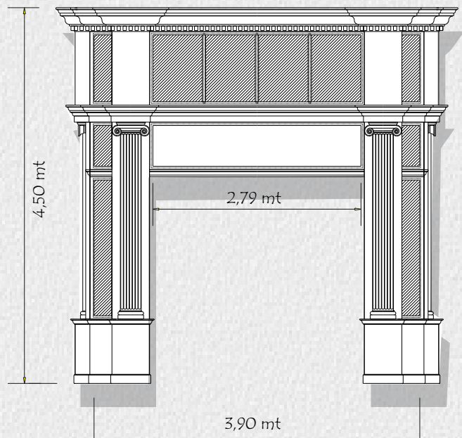
PROSPETTO
